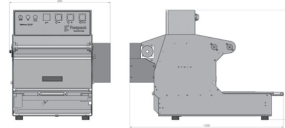
LAY-OUT ReeTray 25 FGT / VGT
